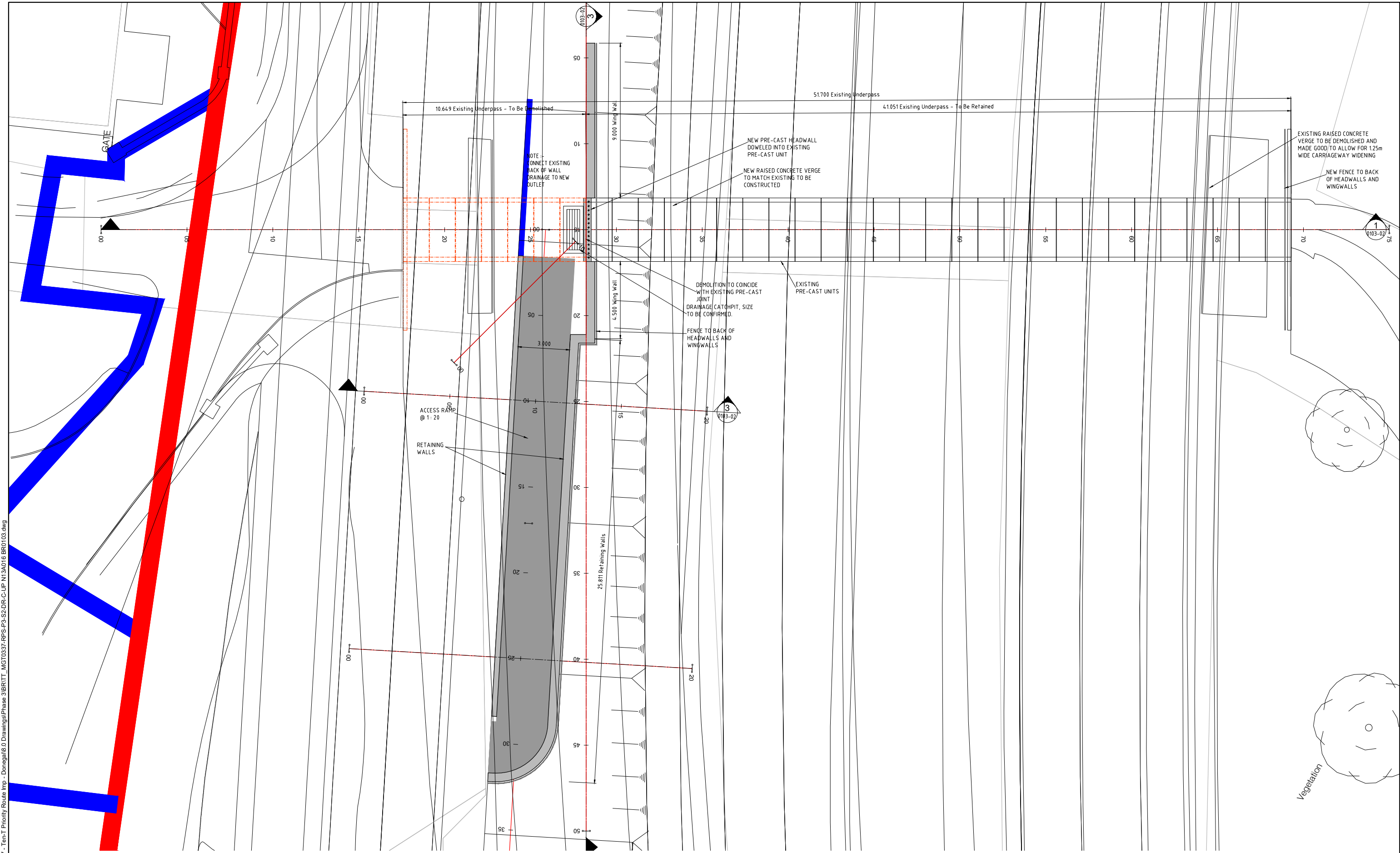
PLAN LAYOUT (Scale 1 : 100)
